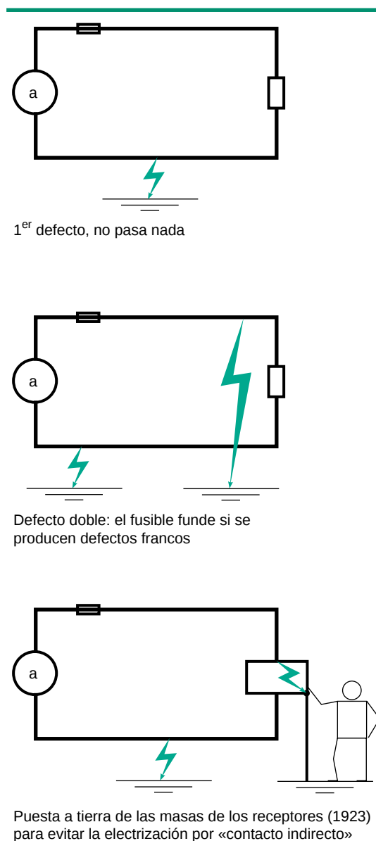
Fig. 2: Inicialmente, la aparición del neutro aislado.
