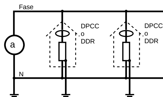
Fig. 4: Neutro a tierra en distribución monofásica.
